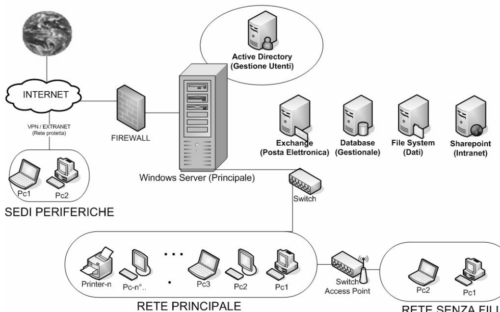
SCHEMA DI RETE
